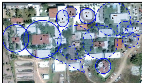
Distribución de antenas y equipos para el servicio de red inalámbrica en los campus Norte. y Manzanillo- El Naranj
